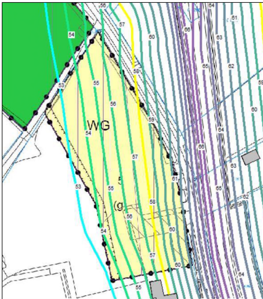
Figuur 4.4 Zilverbaan 10,5 meter contour.
