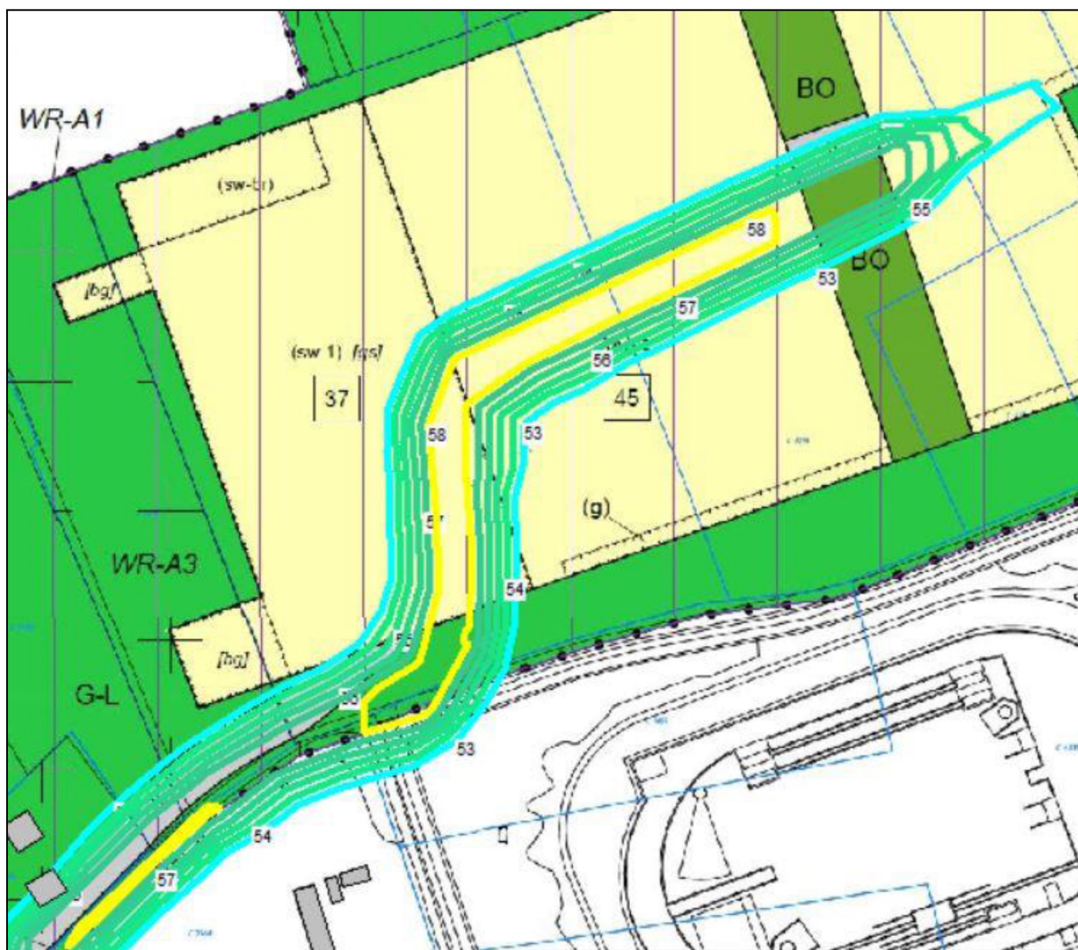
Figuur 4.16 Kransackerweg 4,5 meter contour.
