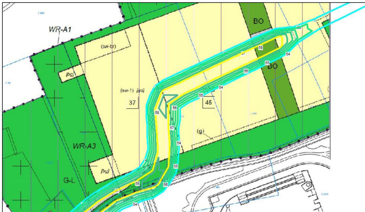
Figuur 4.15 Kransackerweg 1,5 meter contour.
