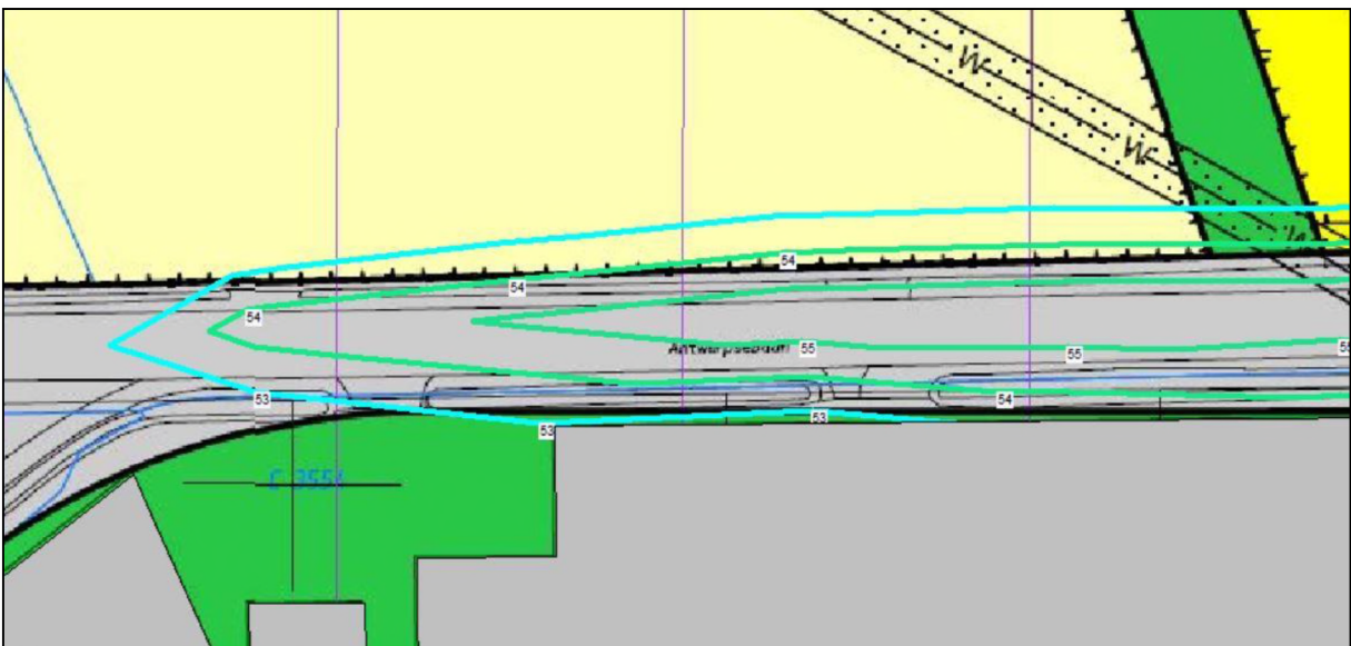
Figuur 4.11 Antwerpsebaan 10,5 meter contour.
