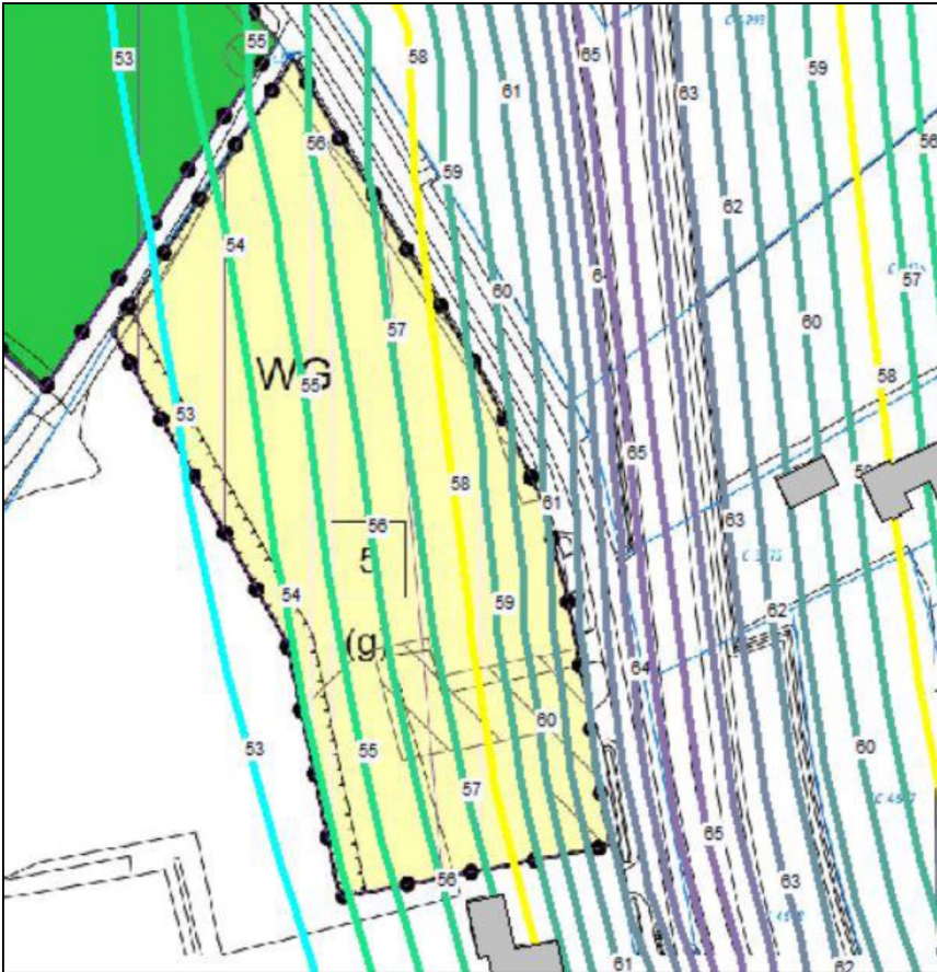
Figuur 4.5 Zilverbaan 13,5 meter contour.
