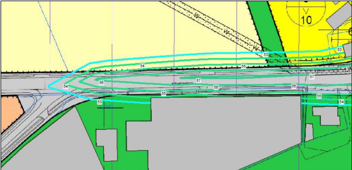
Figuur 4.10 Antwerpsebaan 7,5 meter contour.
