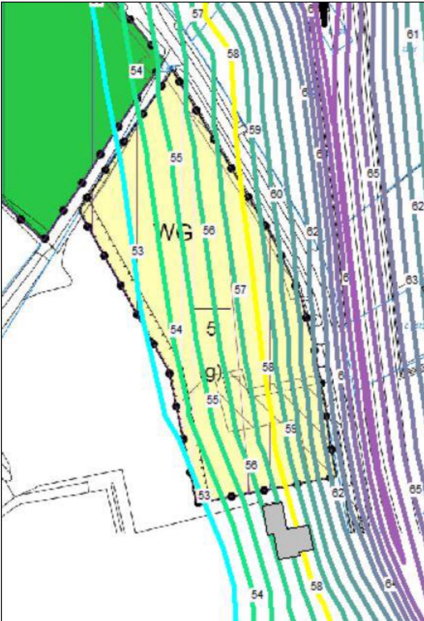
Figuur 4.3 Zilverbaan 7,5 meter contour.
