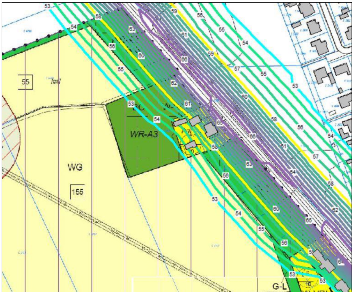
Figuur 4.5 Sondervick 7,5 meter contour.
