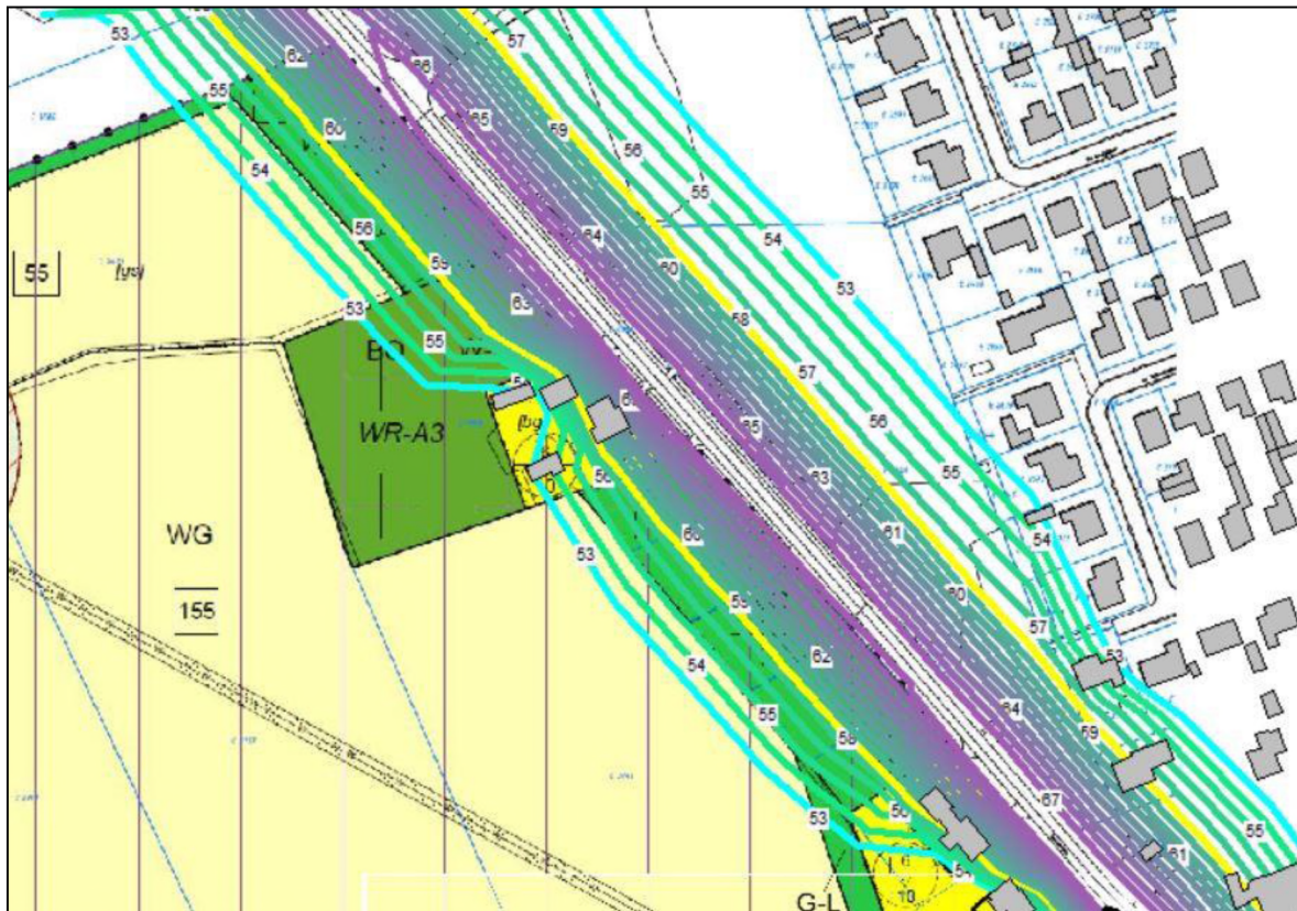
Figuur 4.4 Sondervick 4,5 meter contour.
