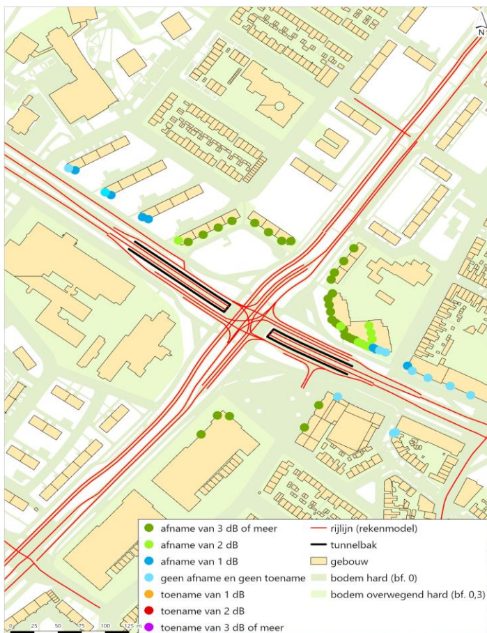
Afbeelding 4.8 geluideffecten van de fysieke wijziging van het verkeersplein (Karel de Grotelaan - Limburglaan)
