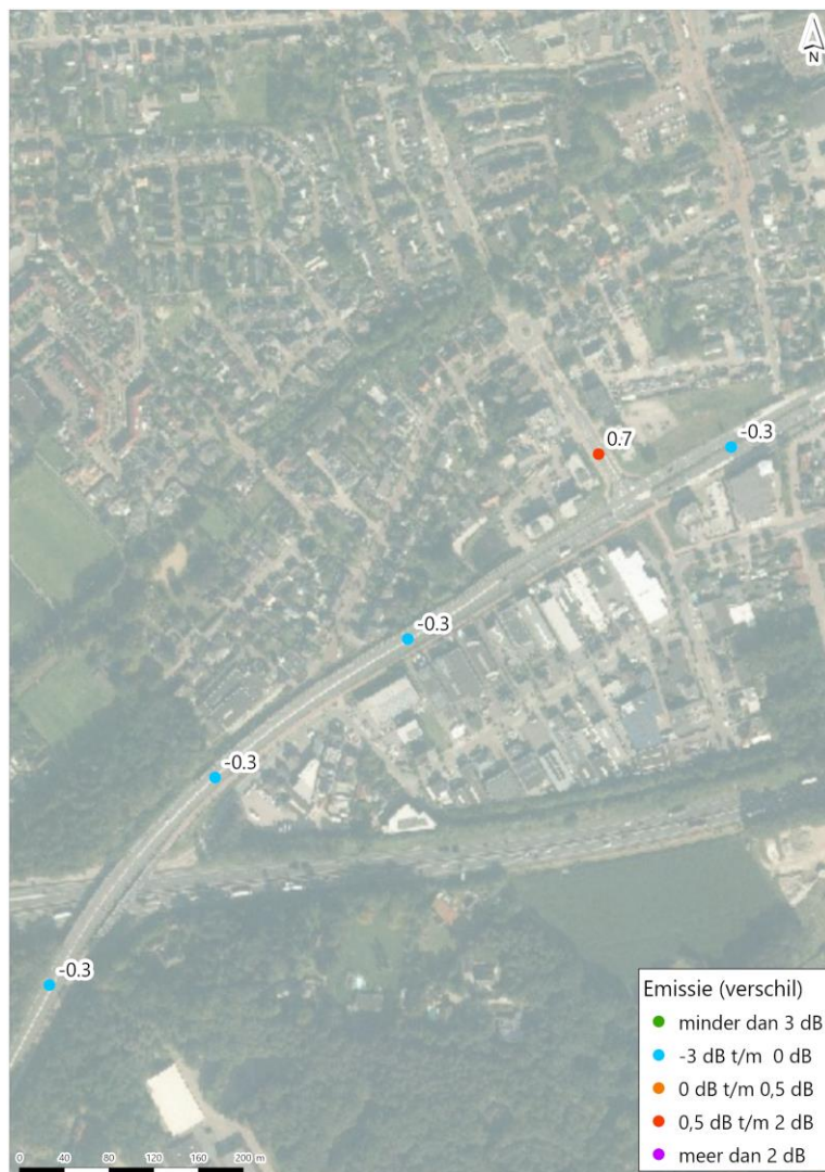
Afbeelding 4.1 Locatie 1 - wegtracé tussen de kruising A67 en de Plank
