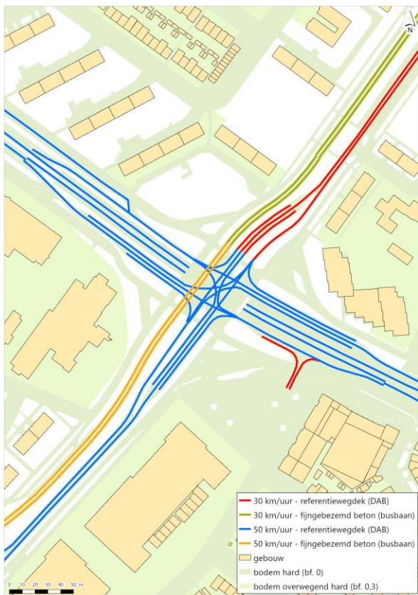
Afbeelding IX.II Toekomstige situatie verkeersplein
