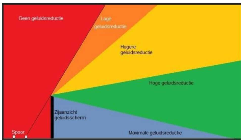
Afbeelding 4.4 Uitleg geluidsschaduw bij schermen langs (spoor-)wegen
