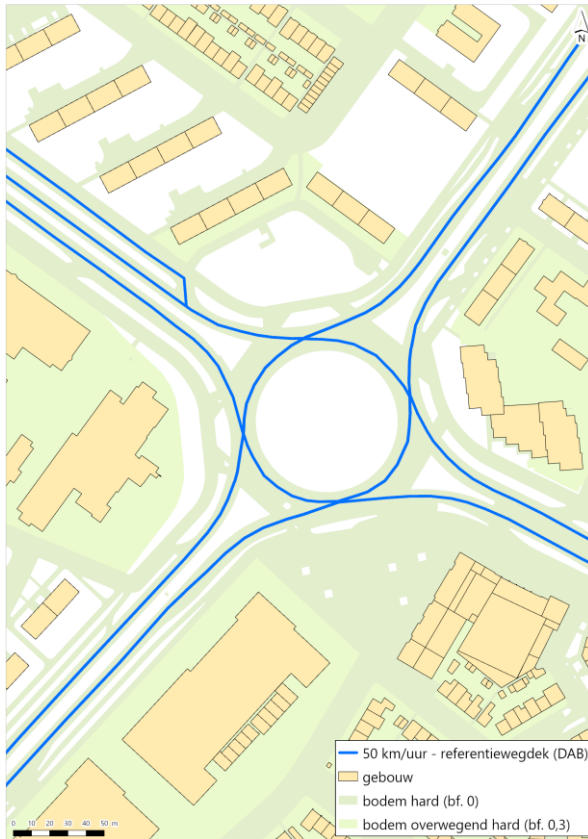
Afbeelding IX. I Huidige situatie verkeersplein
