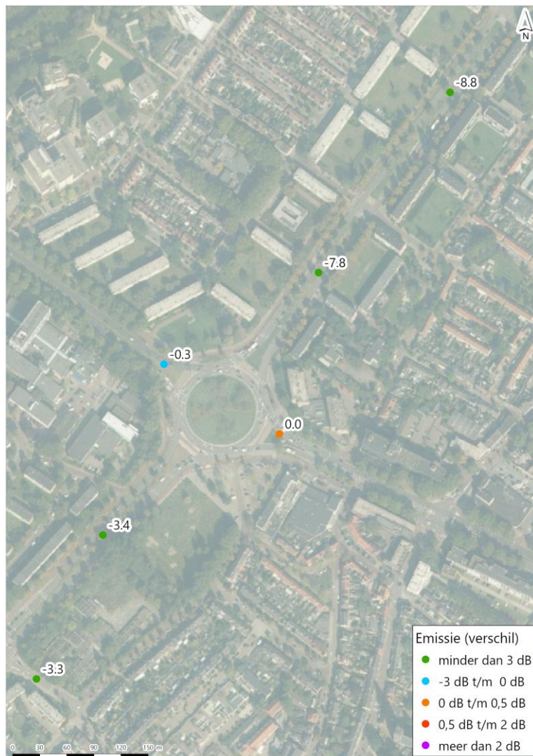
Afbeelding 4.3 Locatie 3 - wegtracé Verkeersplein (Karel de Grotelaan - Limburglaan)
