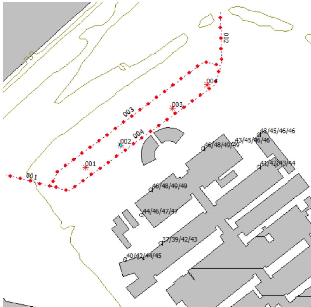
Afbeelding 4.9 Resultaten langtijdgemiddeld beoordelingsniveau - ligging bronlijnen en piekbronnen
