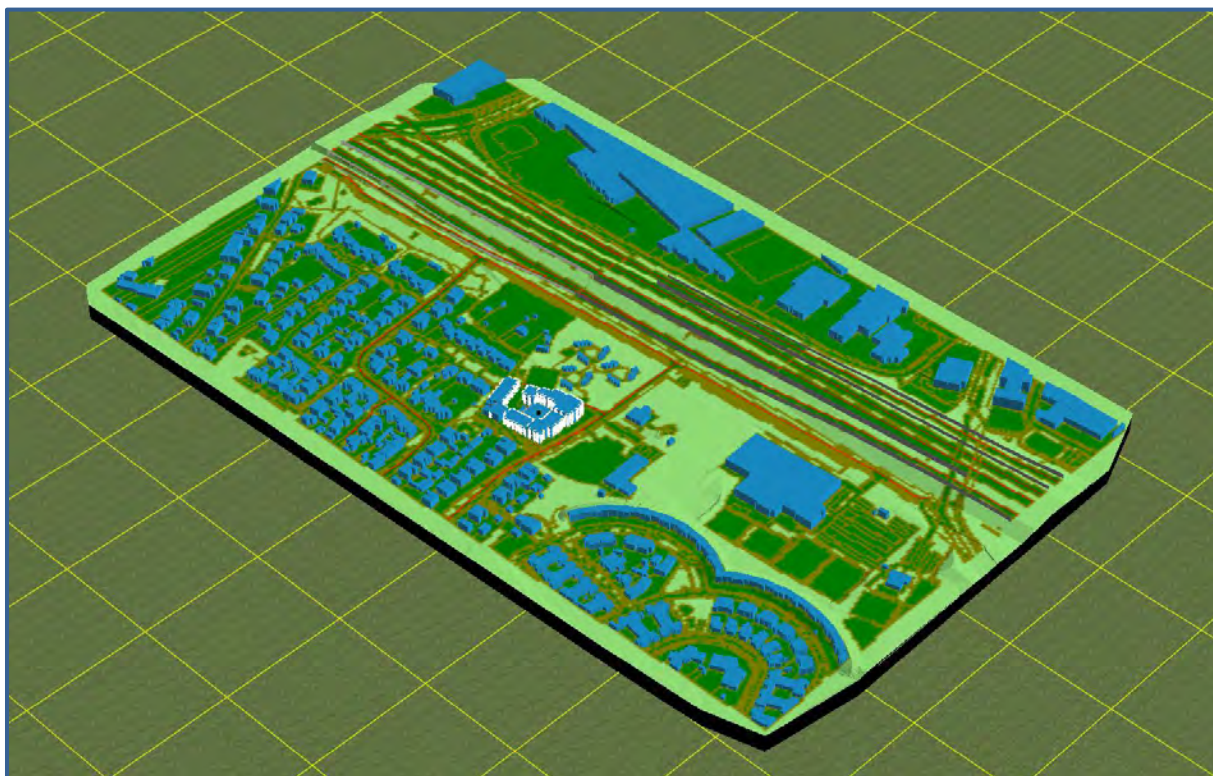
Afbeelding 4. Rekenmodel wegverkeerslawaaï, 3d-weergave (overzicht)
