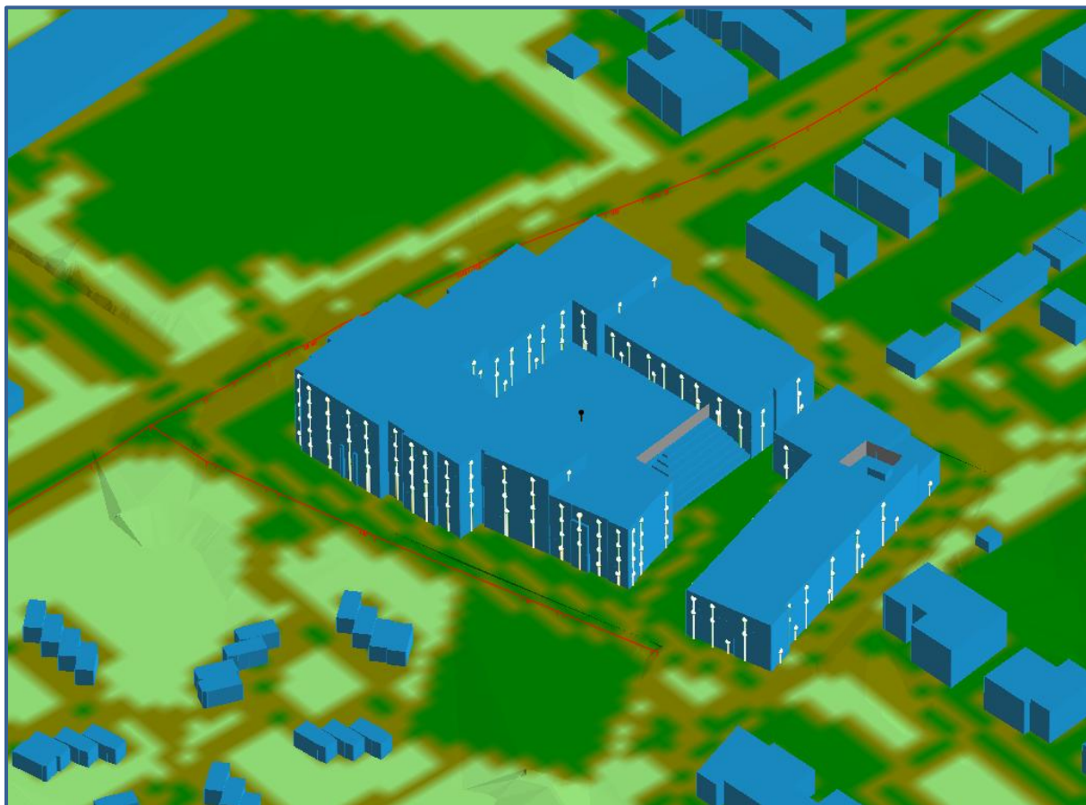
Afbeelding 5. Rekenmodel wegverkeerslawaaï, 3d-weergave (detail)
