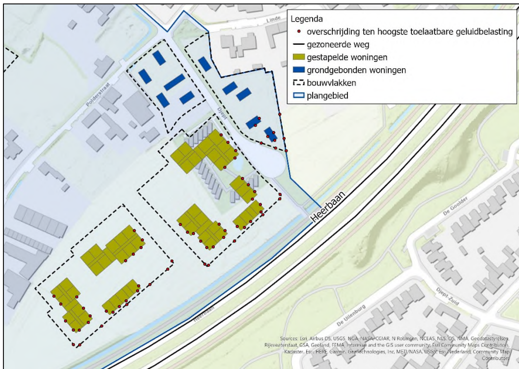
Figuur 4.8 Toetspunten met een overschrijding van de ten hoogste toelaatbare geluidbelasting als gevolg van verkeer op de Heerbaan na toepassing van de voorgestelde bronmaatregel.
