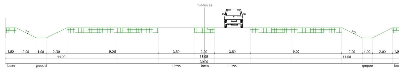
dwarsprofiel 2
