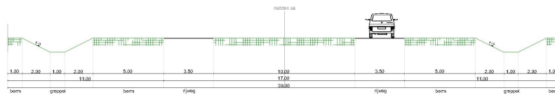
dwarsprofiel 3
