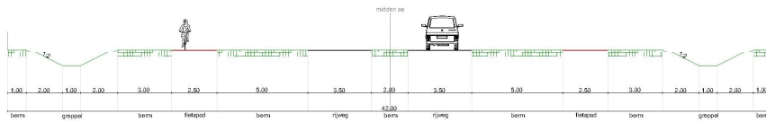
dwarsprofiel 1
